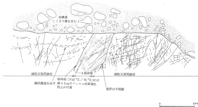
第 3.4.2.4 図 トレンチ地質展開図(その 2) (南東側側壁底部スケッチ)
