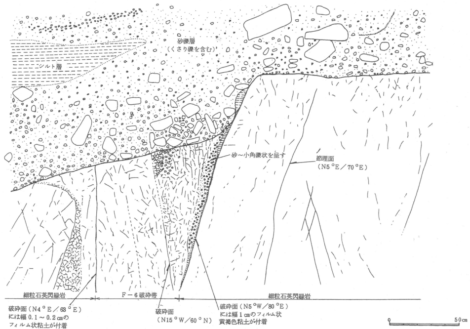
第 3.4.2.4 図 トレンチ地質展開図(その 3) (北西側側壁底部スケッチ)
