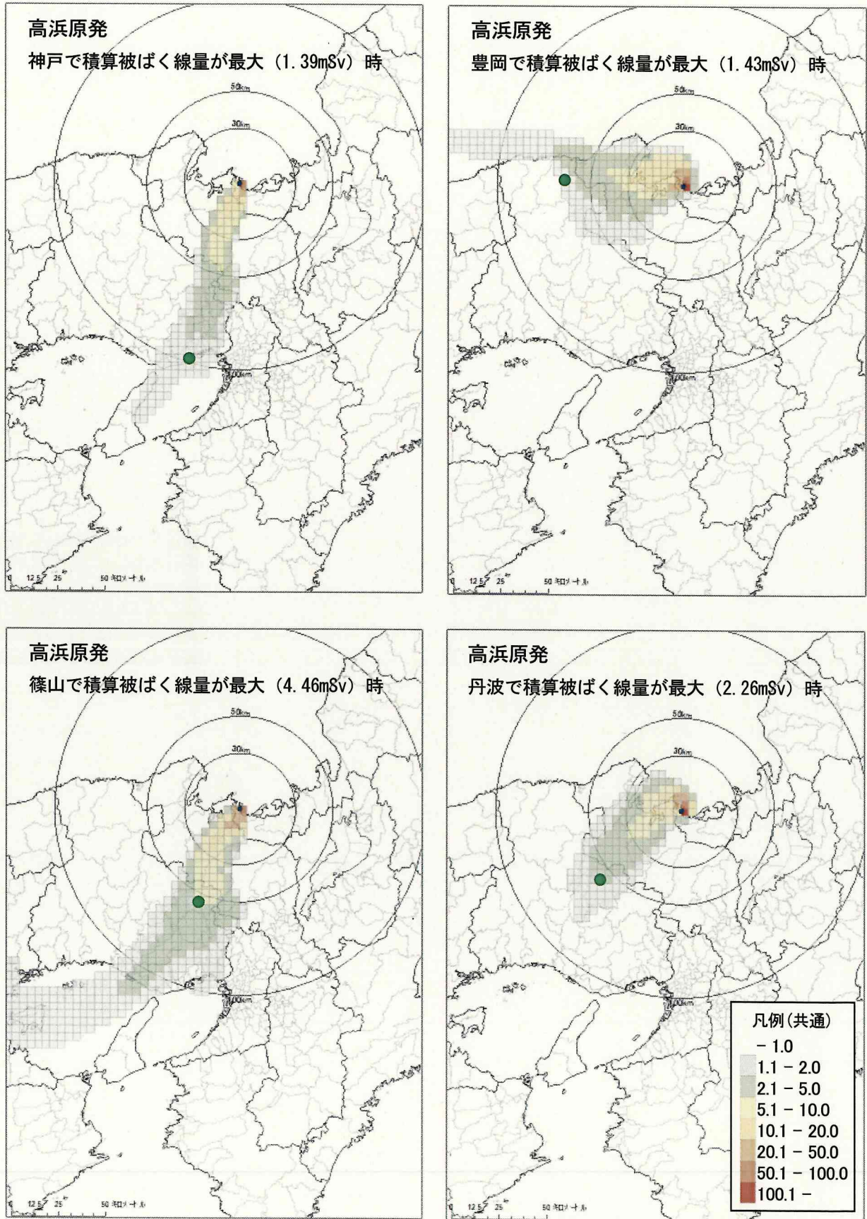
【図2】実効線量
