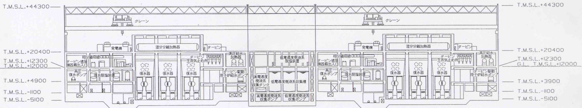
B-B断面図
