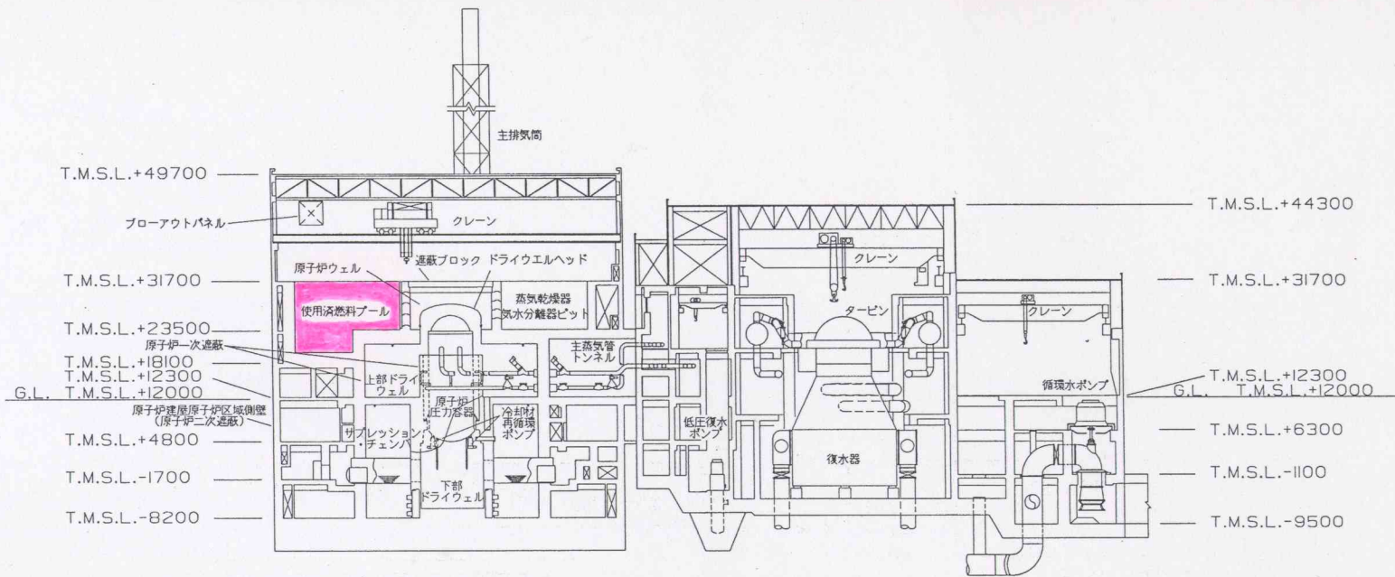
A-A断面図
